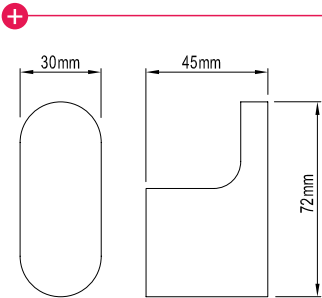
ROBE HOOK (7)620987
