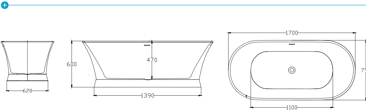
YORK FREESTANDING BATH (7)711724
