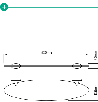
GLASS SHELF (7)620974
