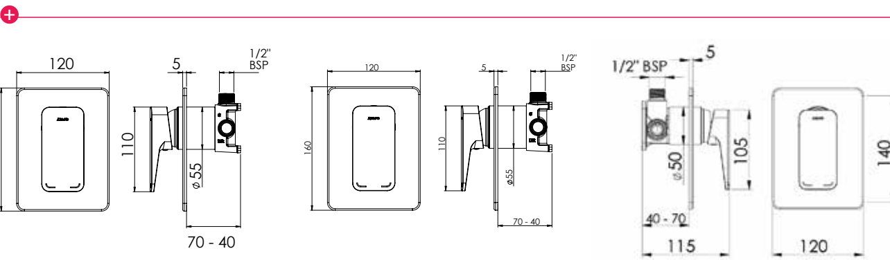
SHOWER MIXER FUSION PLUS (7)706461
